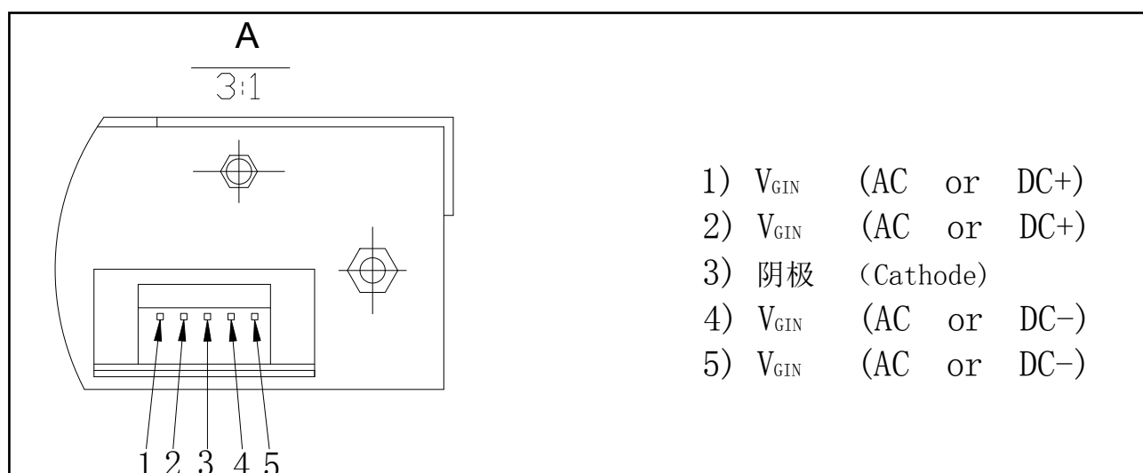
图8. 门极单元电源接口引脚图
