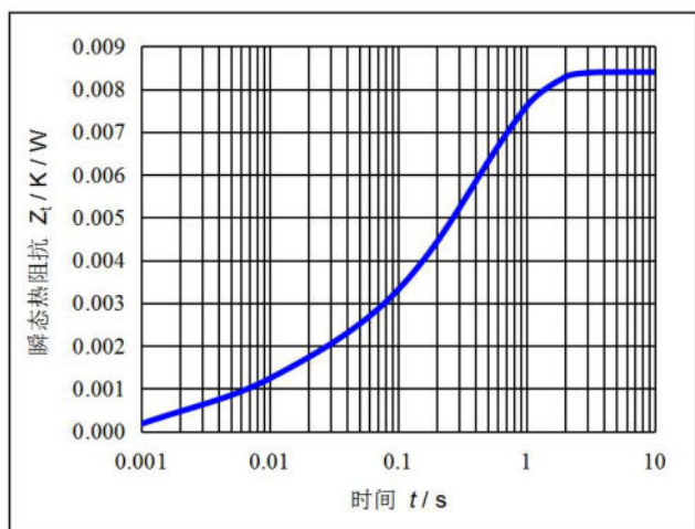
图5. 瞬态热阻抗曲线
